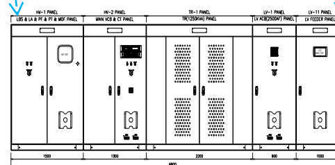
MCBS를 적용한 수배전반
